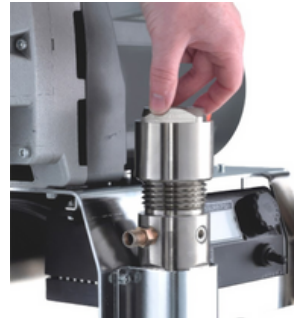
Schnellwechsel-Verteilerfilter
